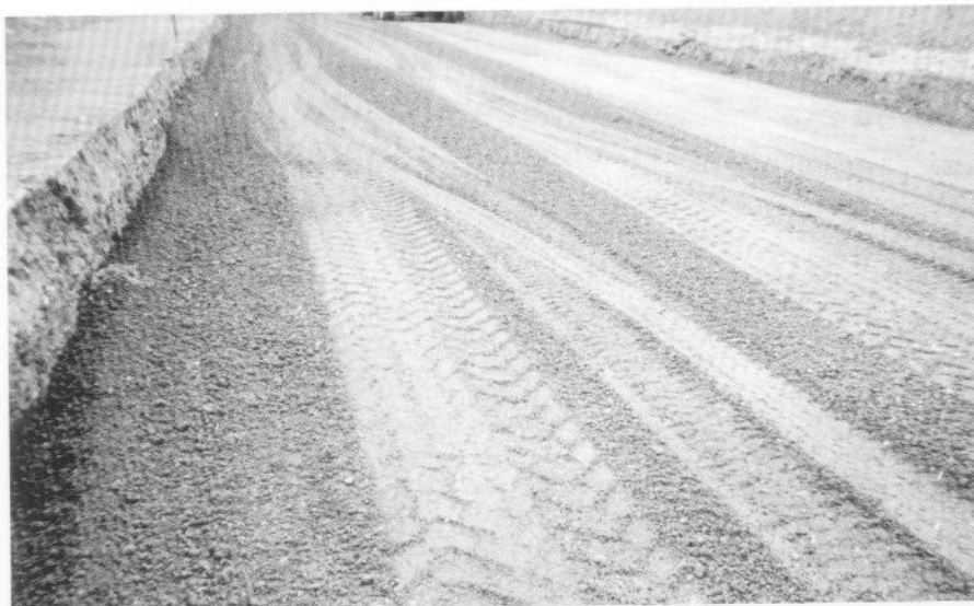
Le mâchefer avant compactage en couche de forme offre une bonne stabilité
