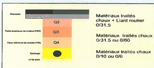
Schéma n°4 : Coupe générale de remblais de tranchées et utilisation des matériaux traités
